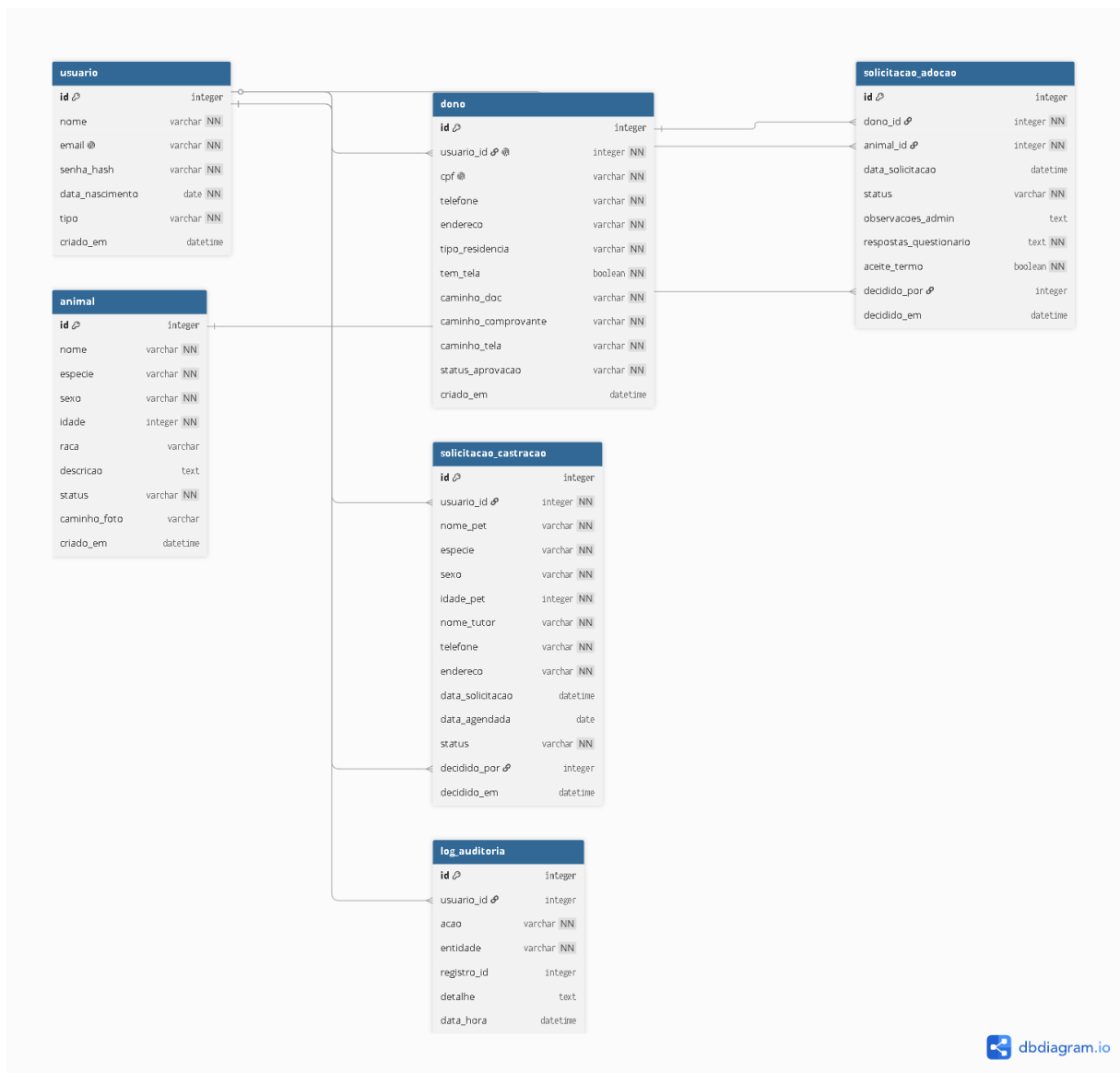
Figura 1 - Diagrama Entidade-Relacionamento, gerado no dbdiagram.io a partir de docs/diagrama_er.dbml
